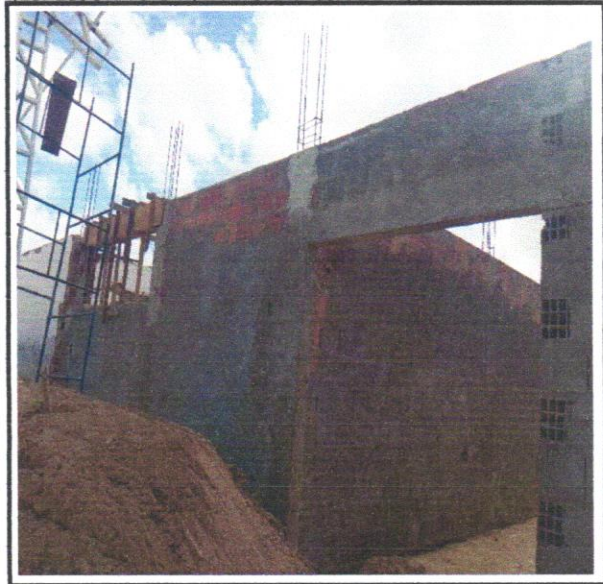
FOTO-14 ALVENARIA DE VEDAÇÃO DE BLOCOS CERÂMICOS FURADOS NA HORIZONTAL DE 9X19X19 CM (ESPESSURA 9 CM) E ARGAMASSA DE ASSENTAMENTO
