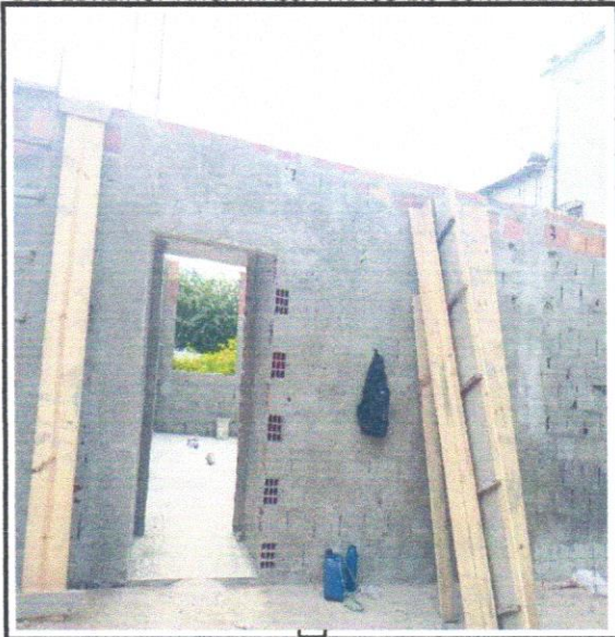
FOTO-13 CHAPISCO APLICADO EM ALVENARIAS E ESTRUTURAS DE CONCRETO INTERNAS, COM COLHER DE PEDREIRO. ARGAMASSA TRAÇO 1:3 COM PREPARO
