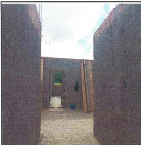
FOTO 15- CHAPISCO APLICADO EM ALVENARIAS E ESTRUTURAS DE CONCRETO INTERNAS, COM COLHER DE PEDREIRO. ARGAMASSA TRAÇO 1:3
